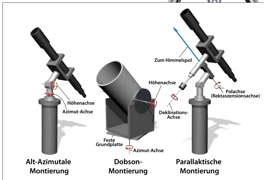
Die beliebtesten Montierungen für Amateur-Teleskope. Astronomy: Roen Kelly
