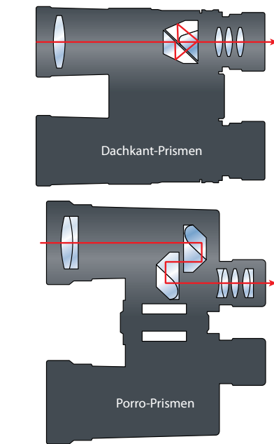
Zwei verschiedene Bauweisen: kompakte Dachkantferngläser oder klassische Porro-Prismen. Astronomy: Roen Kelly
